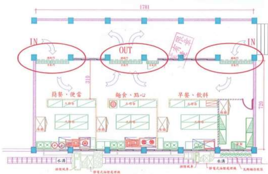
平面圖
